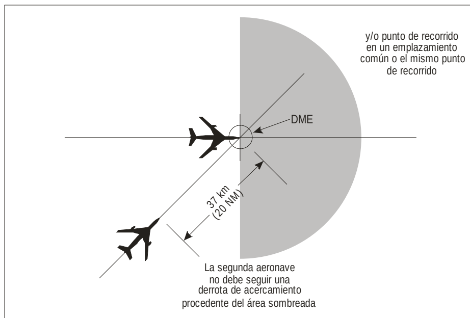
Figura 5-23A. Separación de 37 km (20 NM) basada en DME y/o en GNSS entre aeronaves por derrota que se cruzan y al mismo nivel (véase 5.4.2.3.3.2)
