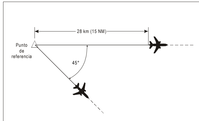
Figura 5-4. Separación utilizando navegación a estima [véase 5.4.1.2.1.2 c)]
