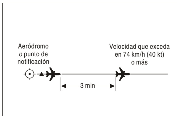
Figura 5-12. Separación de 3 minutos entre aeronaves por la misma derrota y el mismo nivel [véase 5.4.2.2.1.1 d)]
