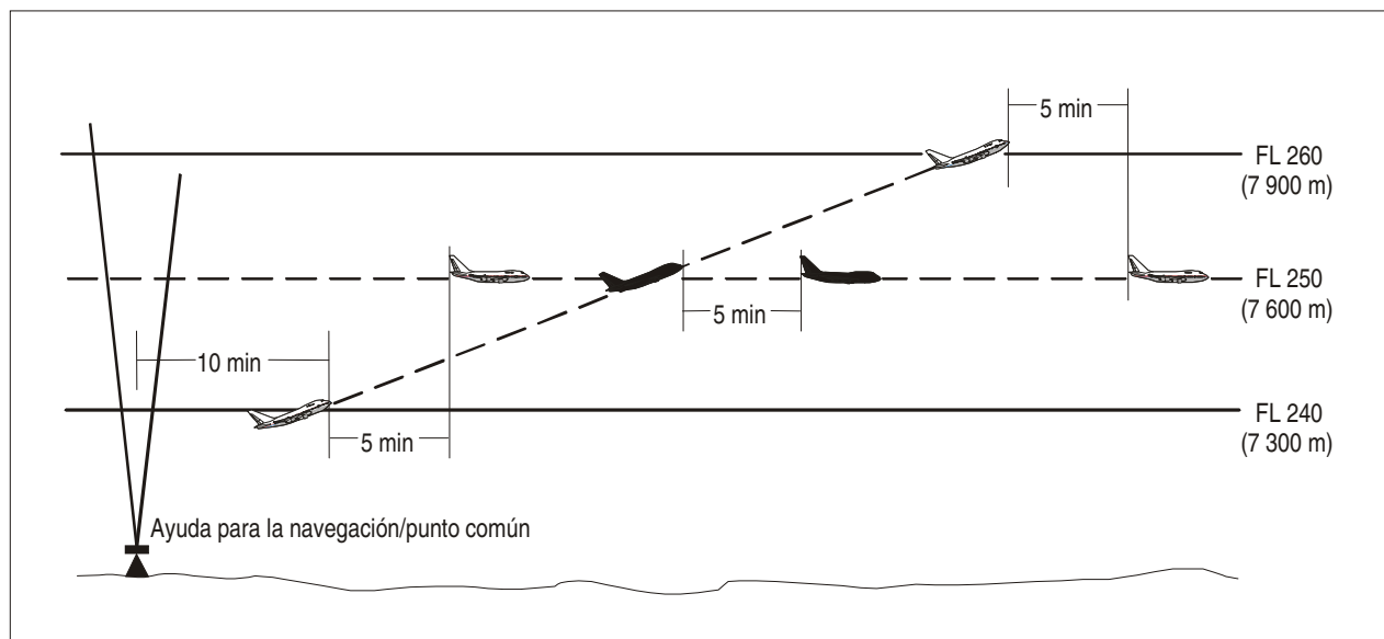
Figura 5-17A. Separación de 5 minutos entre aeronaves que ascienden y por la misma derrota [véase 5.4.2.2.1 c)]
