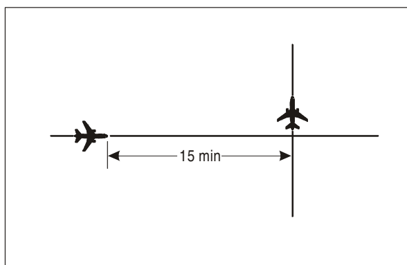
Figura 5-13. Separación de 15 minutos entre aeronaves por derrotas que se cruzan y al mismo nivel [véase 5.4.2.2.1.2 a)]
