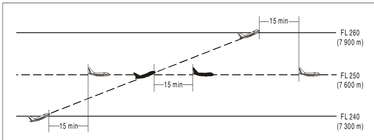
Figura 5-15A. Separación de 15 minutos entre aeronaves que ascienden y por la misma derrota [véase 5.4.2.2.1 a)]
