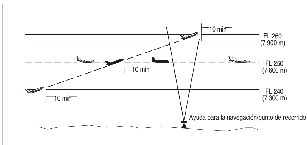
Figura 5-16A. Separación de 10 minutos entre aeronaves que ascienden y por la misma derrota [véase 5.4.2.2.2.1 b)]
