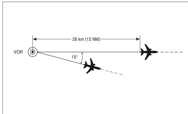
Figura 5-2. Separación utilizando el mismo VOR [véase 5.4.1.2.1.2 a)]
