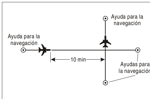
Figura 5-14. Separación de 10 minutos entre aeronaves por derrotas que se cruzan y al mismo nivel [véase 5.4.2.2.1.2 b)]
