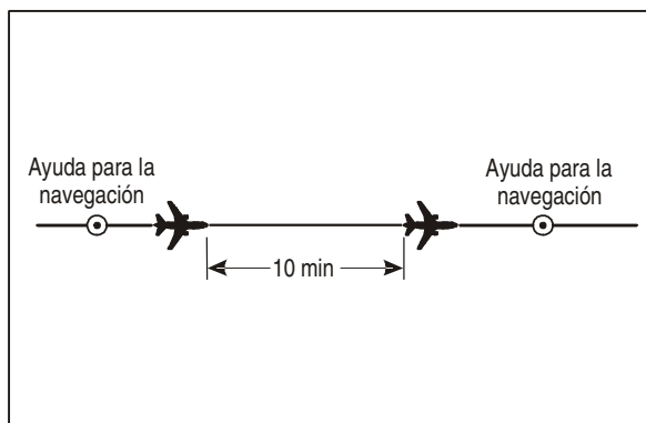
Figura 5-10. Separación de 10 minutos entre aeronaves por la misma derrota y el mismo nivel [véase 5.4.2.2.1.1 b)]
