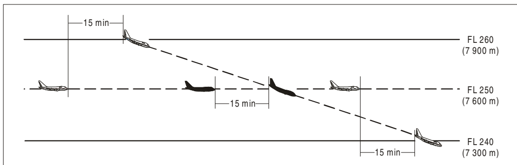
Figura 5-15B. Separación de 15 minutos entre aeronaves que descienden y por la misma derrota [véase 5.4.2.2.2.1 a)]
