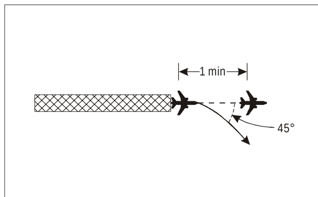
Figura 5-35. Un minuto de separación entre aeronaves que salen y siguen derrota divergentes por lo menos en 45° (véase 5.6.1)
