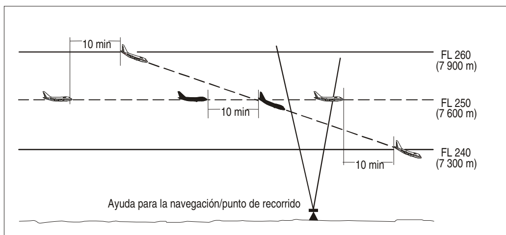
Figura 5-16B. Separación de 10 minutos entre aeronaves que descienden y por la misma derrota [véase 5.4.2.2.2.1 b)]
