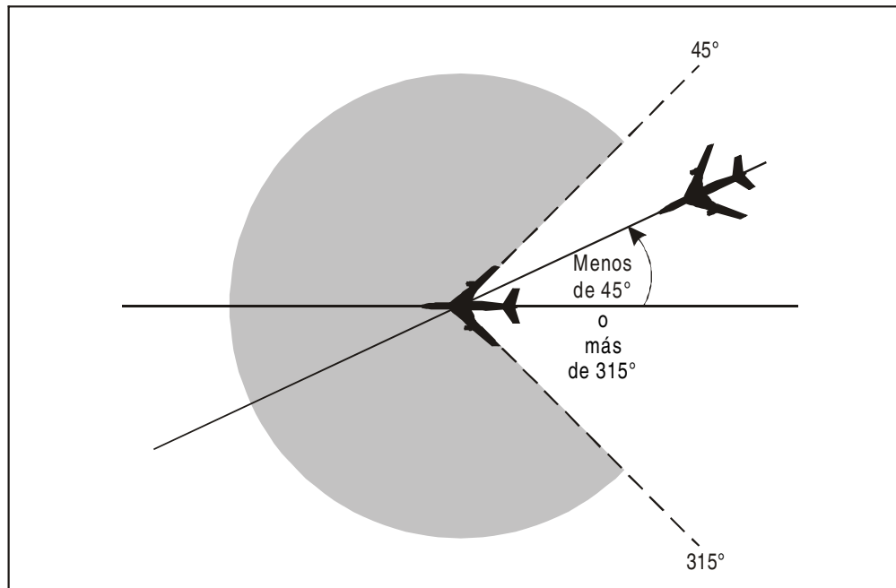
Figura 5-6. Aeronaves por la misma derrota [véase 5.4.2.1.5 a)]
