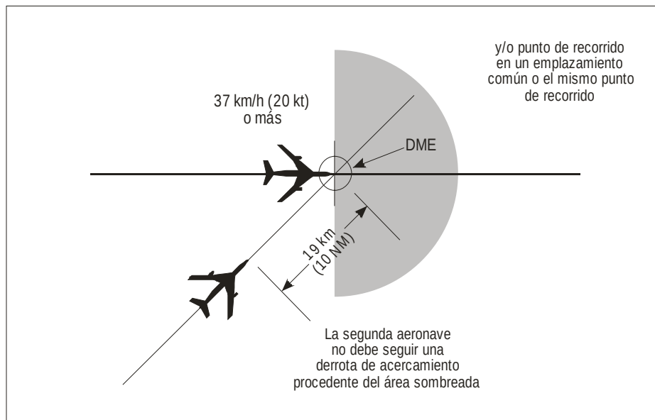
Figura 5-23B. Separación de 19 km (10 NM) basada en DME y/o en GNSS entre aeronaves por derrota que se cruzan y al mismo nivel (véase 5.4.2.3.3.2)
