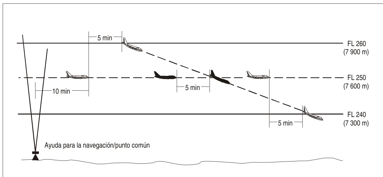
Figura 5-17B. Separación de 5 minutos entre aeronaves que descienden y por la misma derrota [véase 5.4.2.2.1 c)]
