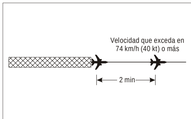
Figura 5-36. Dos minutos de separación entre aeronaves que siguen la misma derrota (véase 5.6.2)
