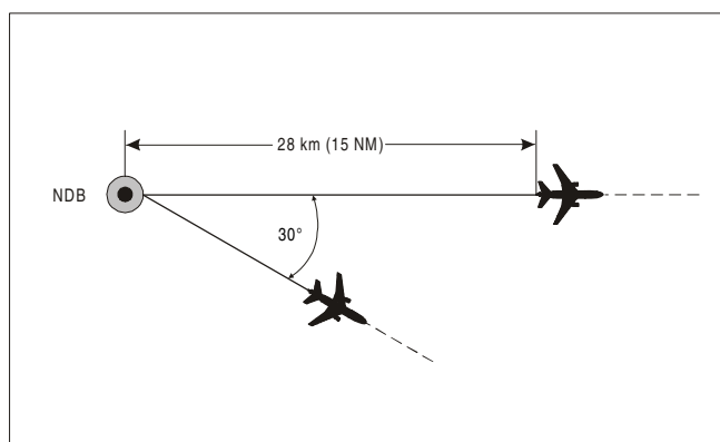
Figura 5-3. Separación utilizando el mismo NDB [véase 5.4.1.2.1.2 b)]
