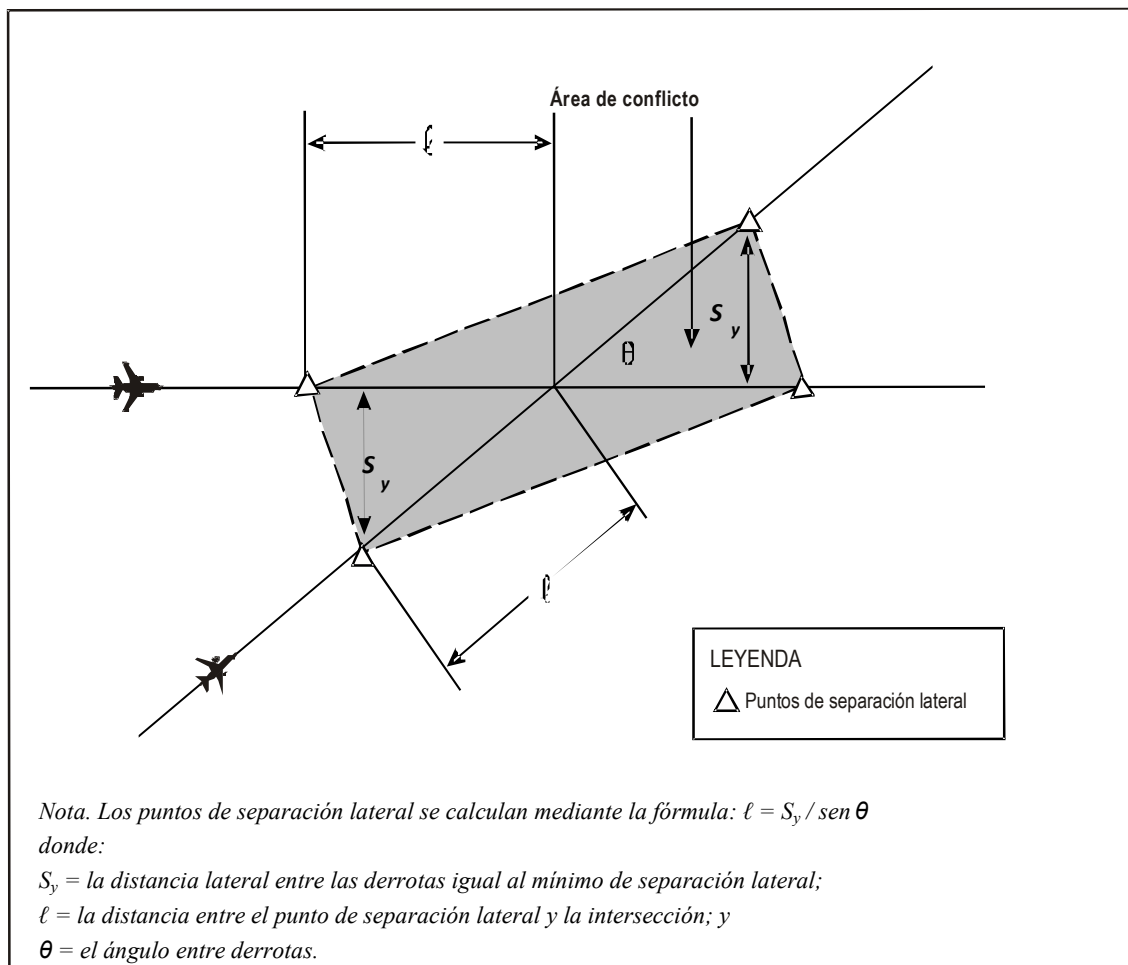
Figura 5-5. Puntos de separación lateral y el área de conflicto (véase 5.4.1.2.1.5.1)
